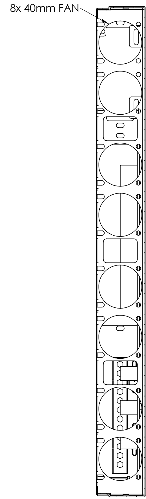
PRZEKRÓJ C-C
