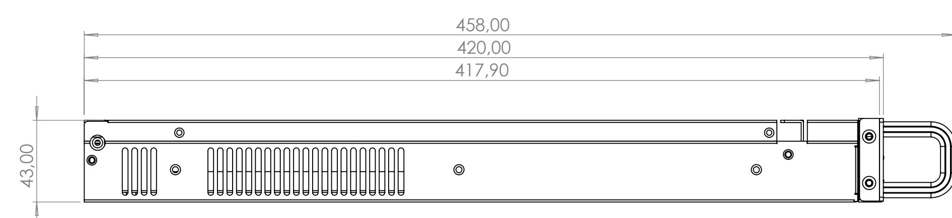
PRZEKRÓJ A-A
